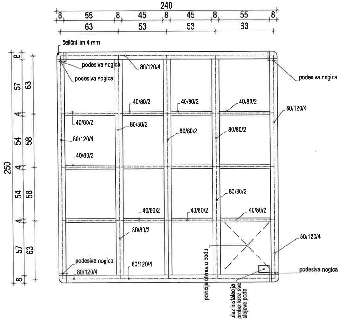
Podna nosiva konstrukcija kontrolne kućice - CARINA
